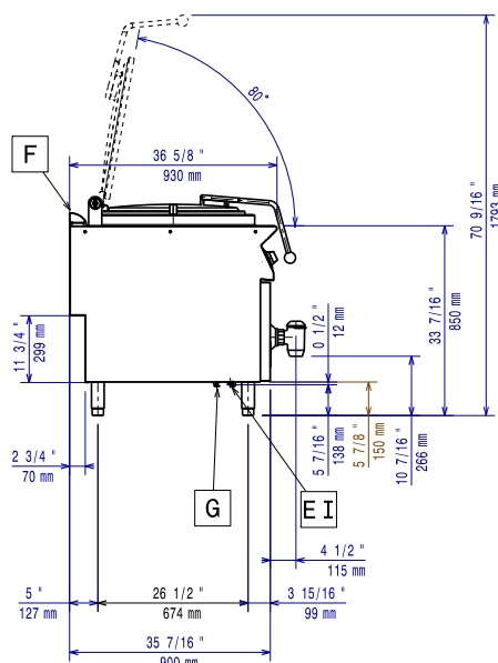
Zij aanzicht
